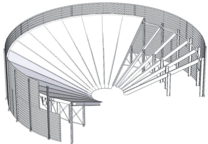
Belüftungskonus
