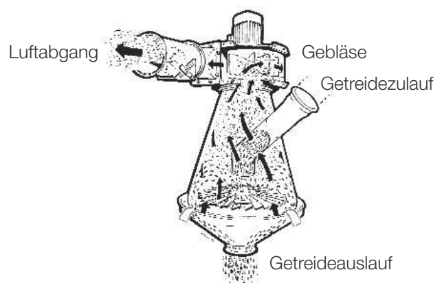
Funktionsprinzip
