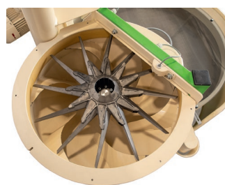
Schleuderrad
